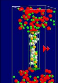
Nanopore DNA
