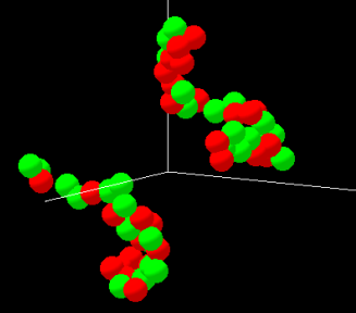
Poly-ampholyte
